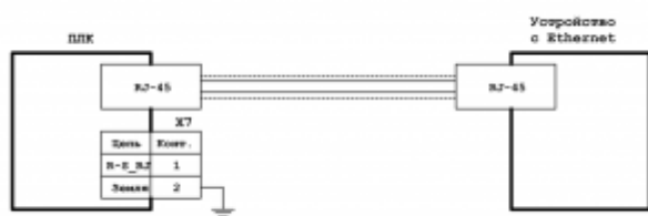
Схема подключения экранированной линии Ethernet
